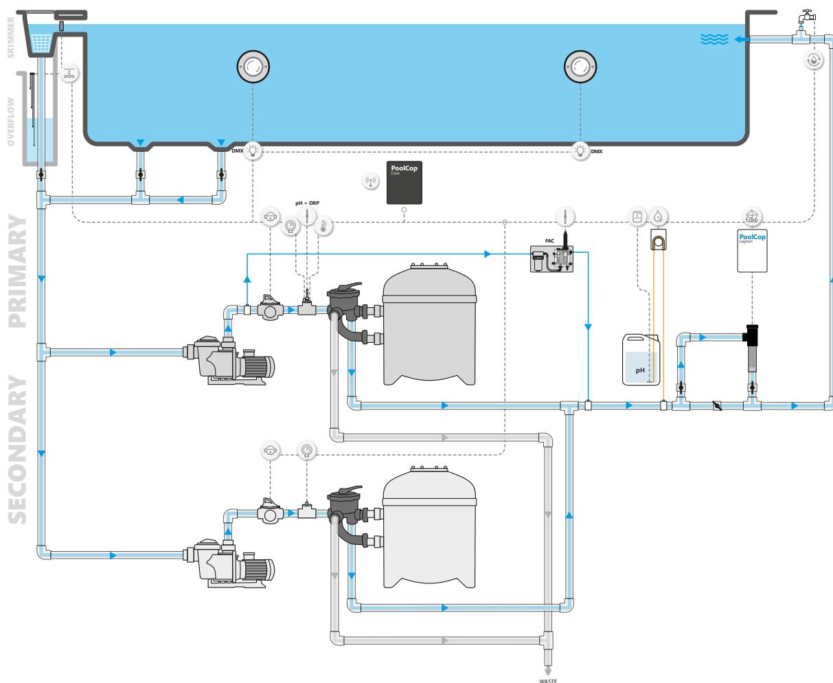
POOLCOP CORE - DEUX POMPES AVEC ACQUISITION DE DONNÉES & DÉSINFECTION AU SEL
