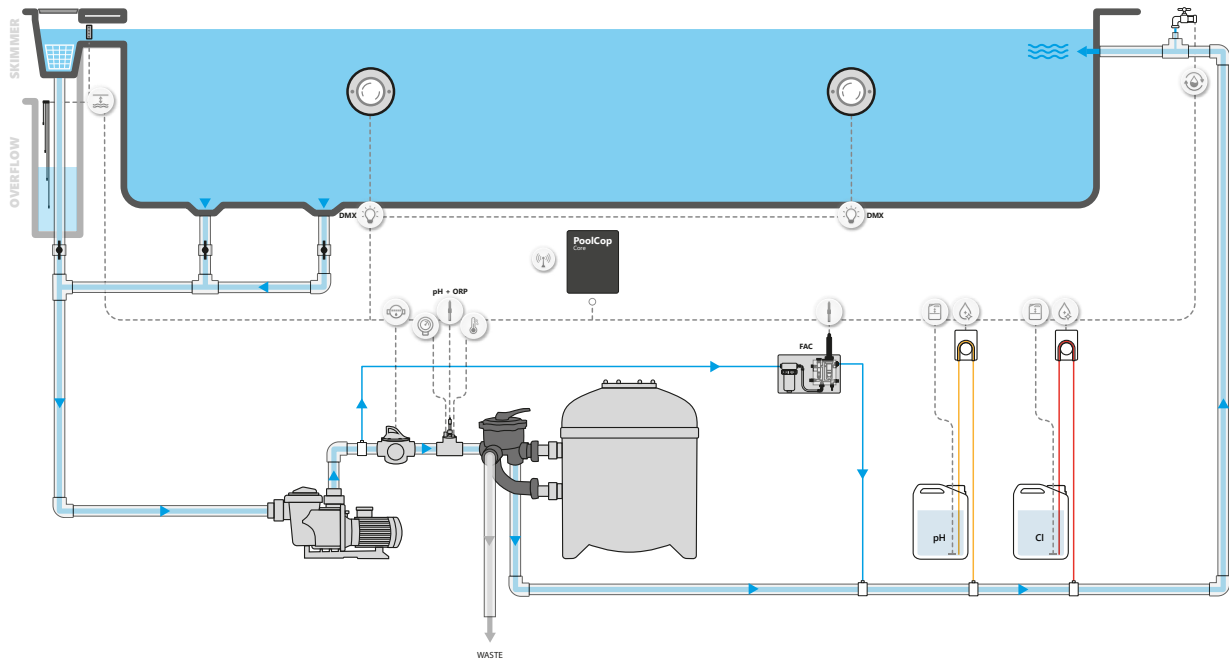
POOLCOP CORE - POMPE UNIQUE AVEC ACQUISITION DE DONNÉES & DÉSINFECTION AU CHLORE
