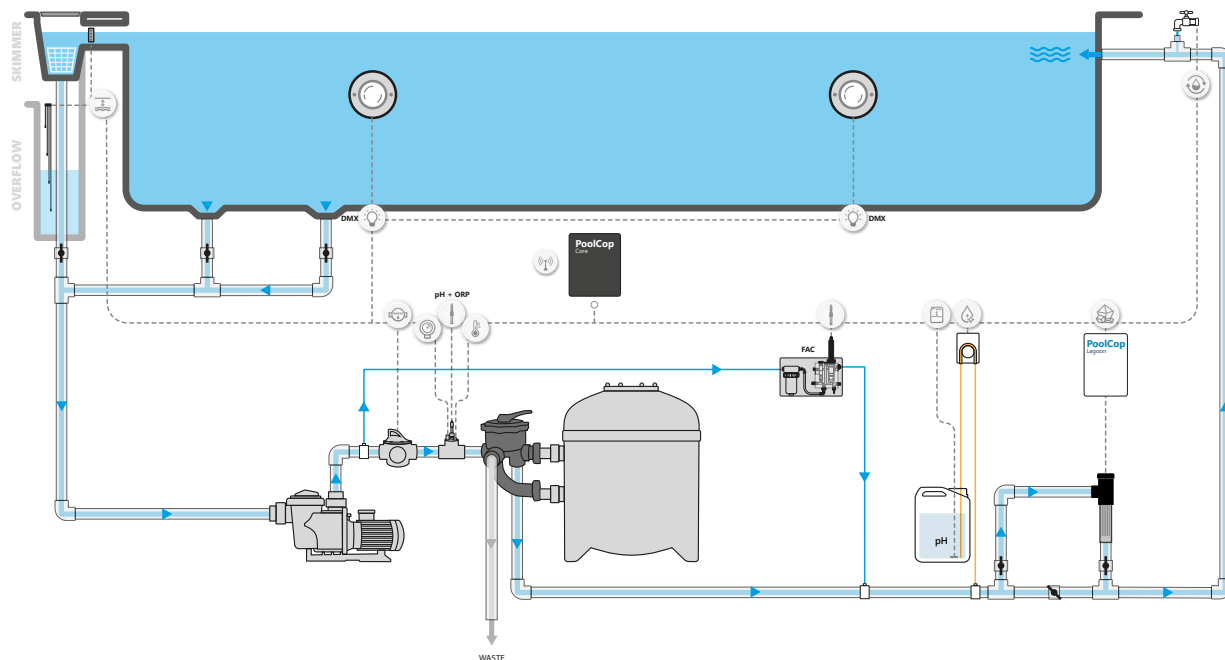
POOLCOP CORE - POMPE UNIQUE AVEC ACQUISITION DE DONNÉES & DÉSINFECTION AU SEL
