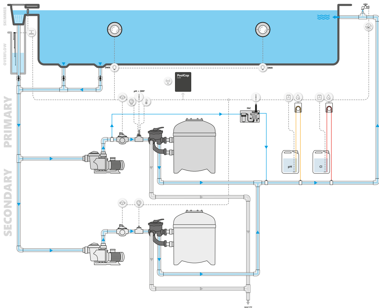
POOLCOP CORE - DEUX POMPES AVEC ACQUISITION DE DONNÉES & DÉSINFECTION AU CHLORE
